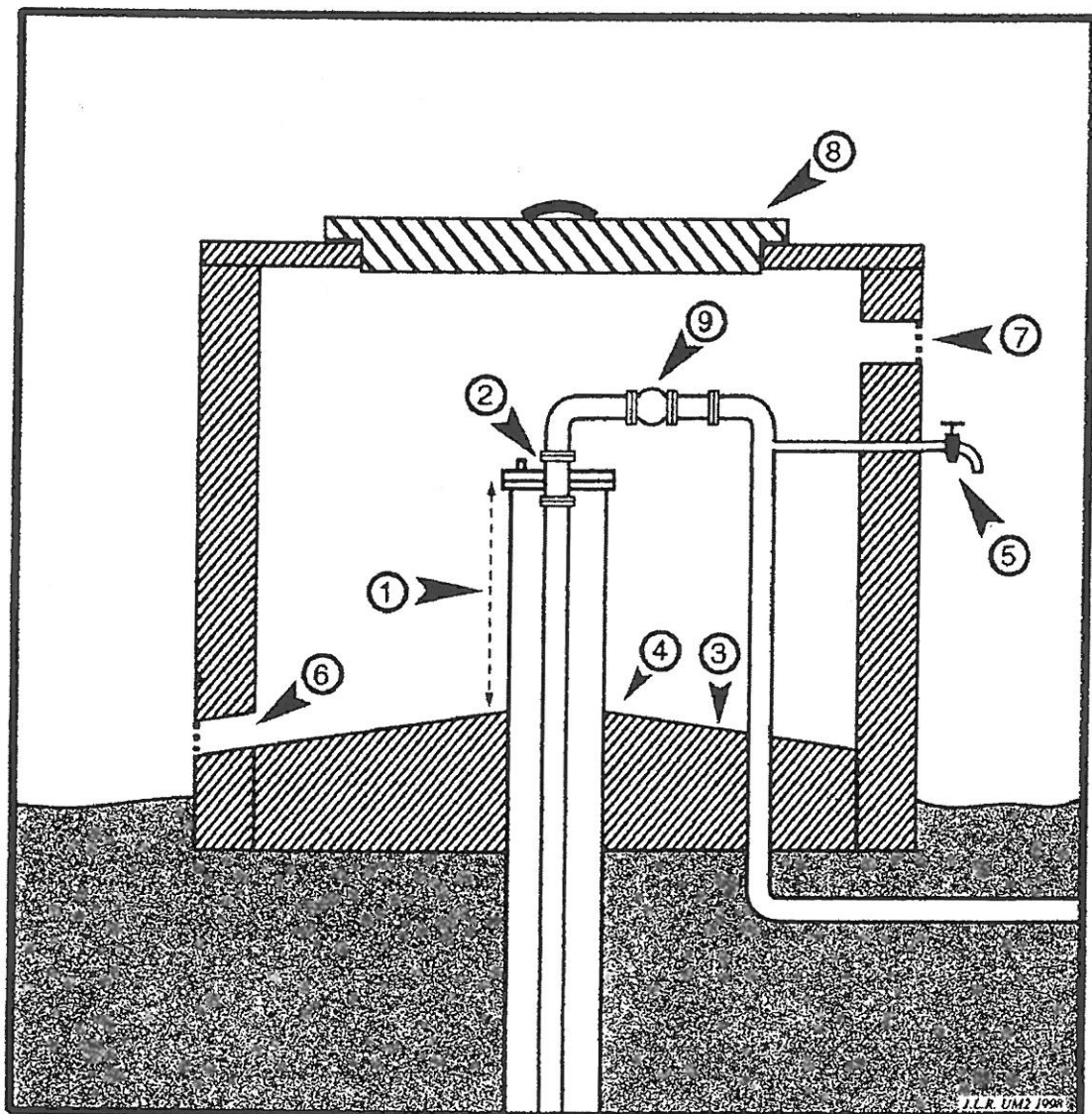
PRINCIPE D'AMÉNAGEMENT D'UNE TÊTE DE FORAGE AEP
